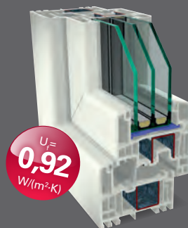
Schmalere Rahmen mit Flügel und bestätigter ift-Passivhaustauglichkeit
