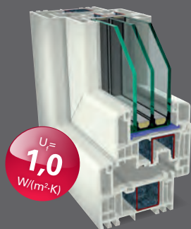
Schmalere Rahmen mit Flügel
